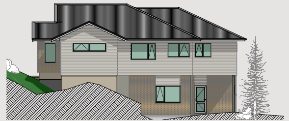
ELEVATION 2
