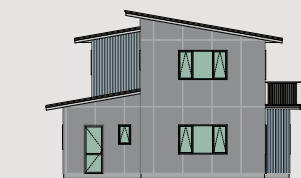
ELEVATION 3
